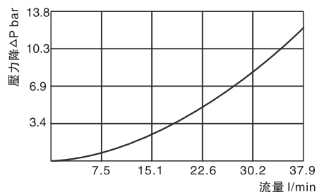
■ 曲綫圖 測試條件：油温：T=50°C，粘度：35cst
