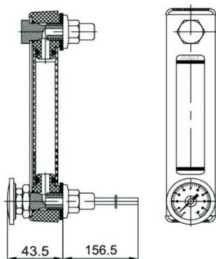
G 温度表型 Type G: Temperature gauge
