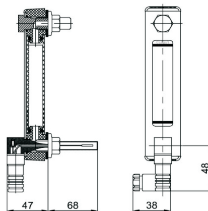
T 温度开关型 Type T: Thermo switch
