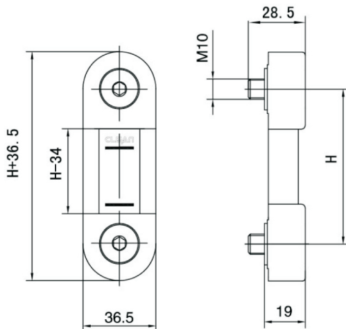
B型 Type B
