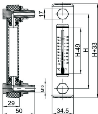
M 温度计型 Type M: Temperature meter
